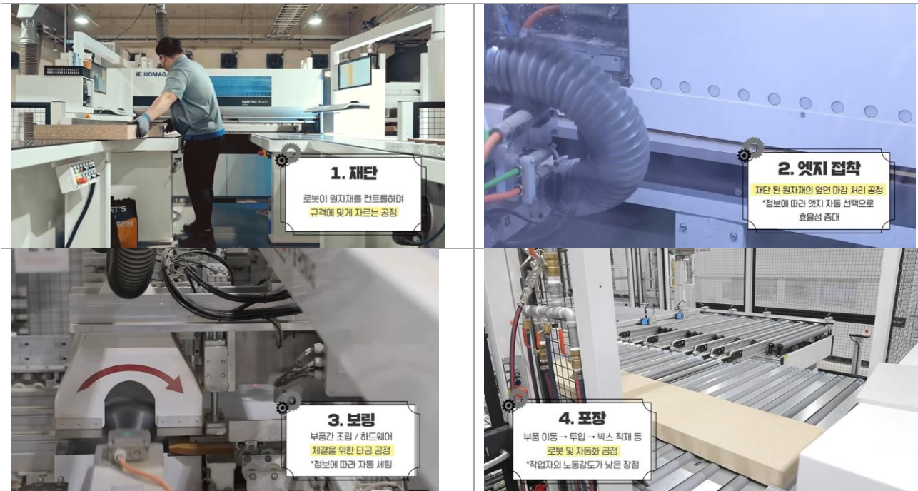
도표 2. 가구 제조 공정 순서 재단 - 엿지처리 - 보링 - 포장
